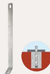
FERRURE DE SELLEMENT AU SOL
